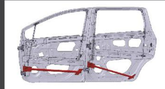
SIDE DOOR IMPACT BEAM ความปลอดภัยที่ครบถ้วนครอบคลุมบริเวณแผงประตู เพื่อลดแรงปะทะจากด้านข้างให้กับผู้โดยสารในกรณีเกิดอุบัติเหตุ
